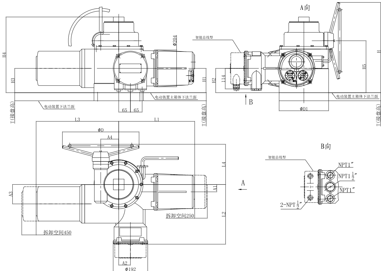
IMC100~300系列外形尺寸
